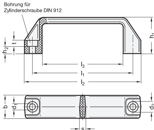
Ausführung ESD
