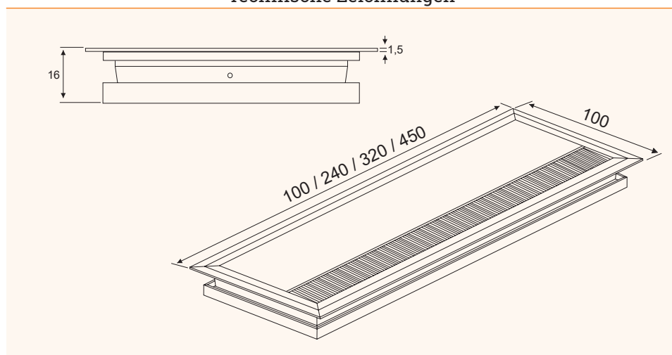
Technische Zeichnungen
