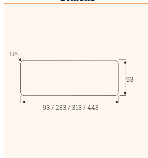
Bohrbild
